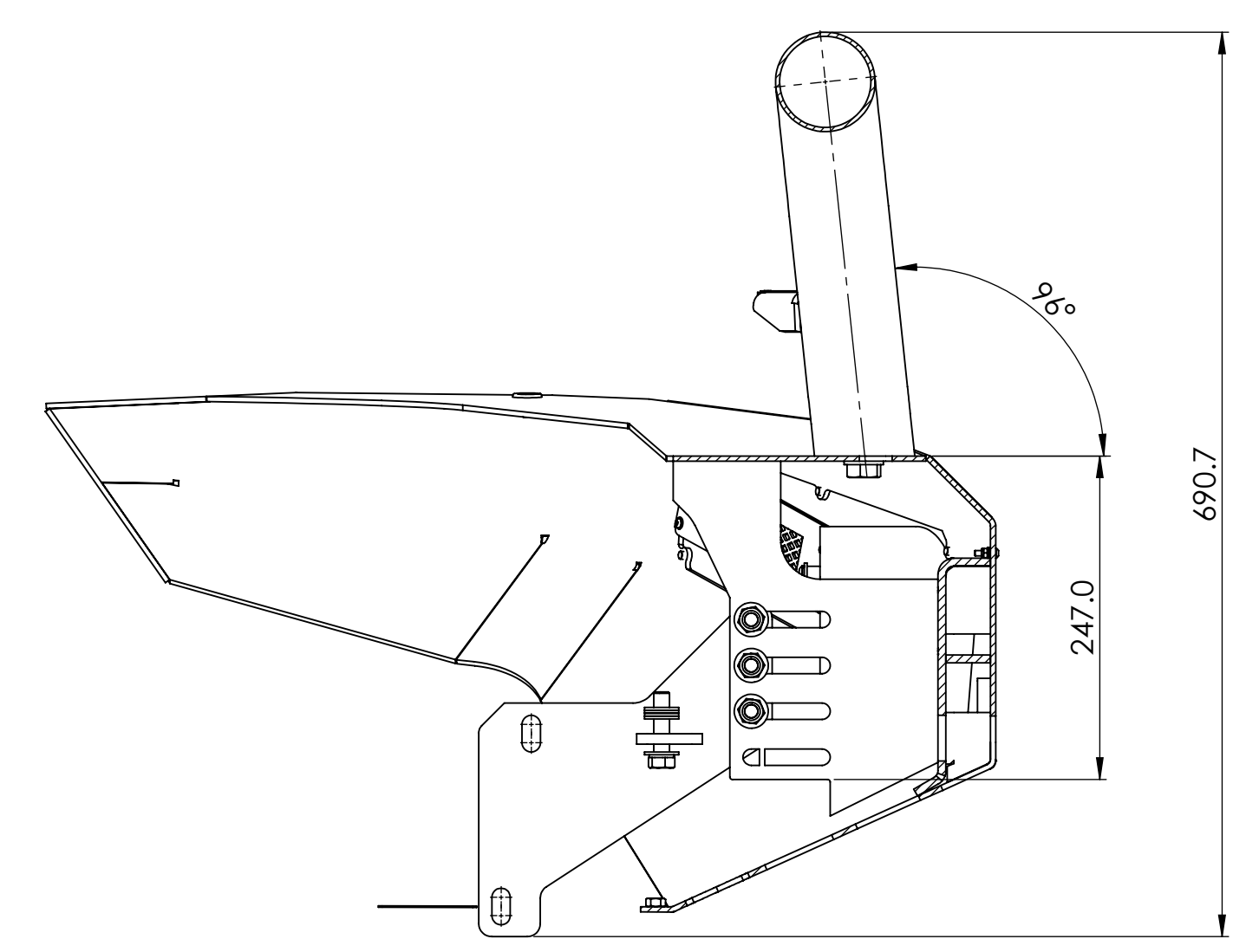
SECTION A-A
